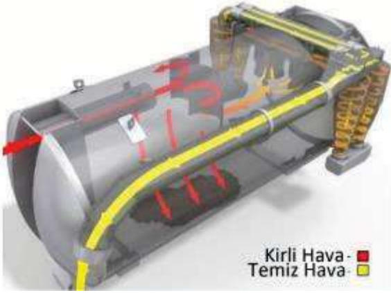
Geniş atık tankı
