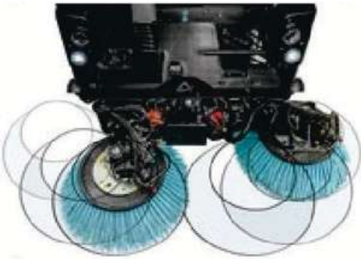
Hem itilir hem çekilir tip fırça sistemi
